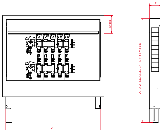
Colector ALB ULTRACOMPACTO 2+3 en caja metálica
