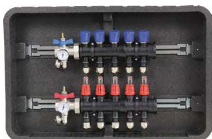
Incluye soportes PA-SOP-CALB
