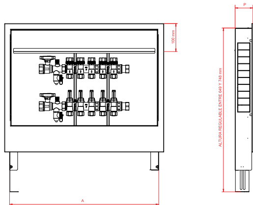
Colector ALB caudalímetro caja metálica
