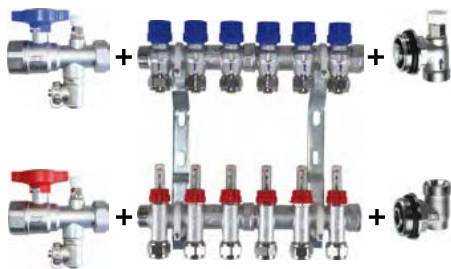
Configuración con válvulas de corte a la izquierda
