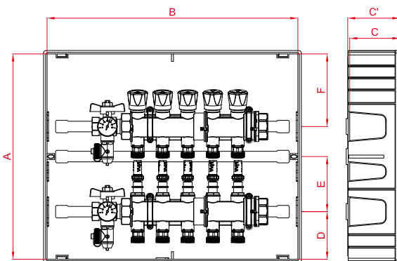
Colector ALB ULTRACOMPACTO 2+3 en caja plástico
