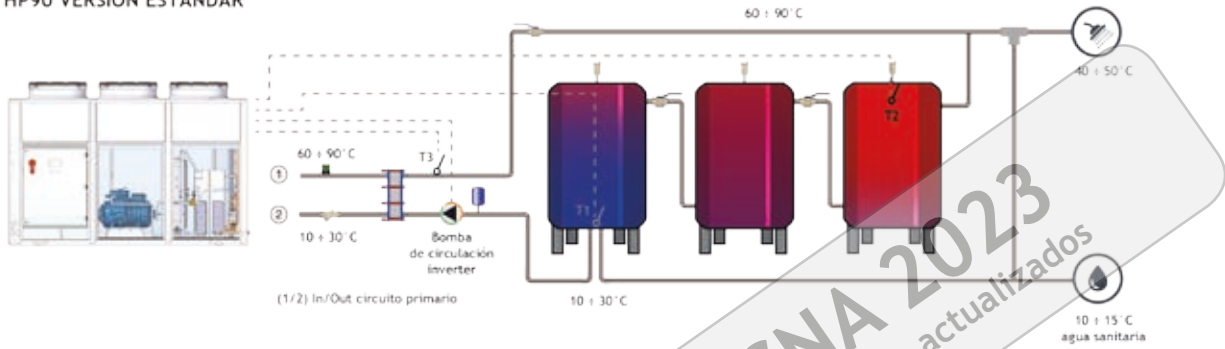
HP90 RECUPERACION DE FRIO
