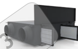
Filtros F7 + HEPA H13 en VMC doble flujo
