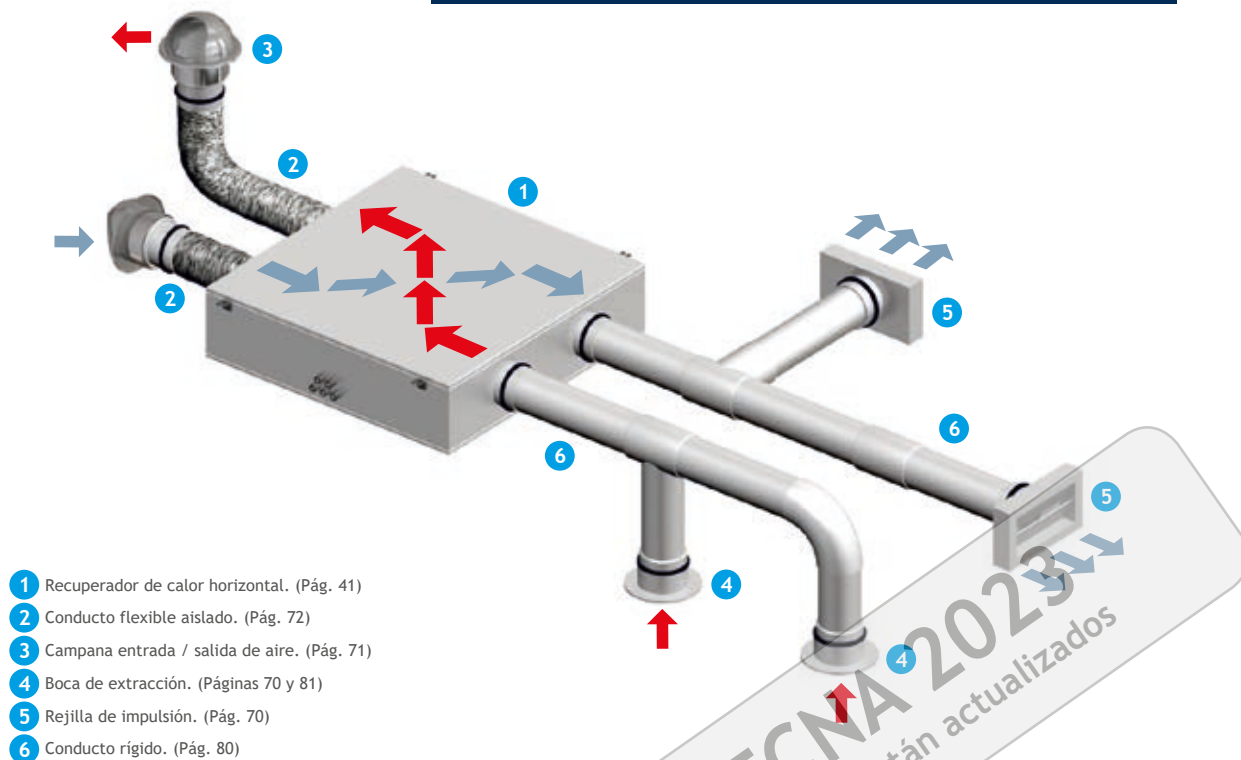
ESQUEMA TIPO VIVIENDA COLECTIVA CON CONDUCTO RÍGIDO
