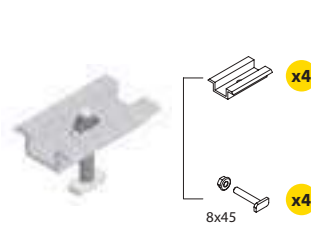
Grapa intermedia con tornillo
