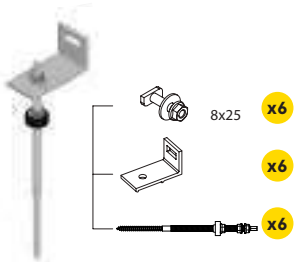
Anclaje pasateja 10x250 con pletina y tornillo
