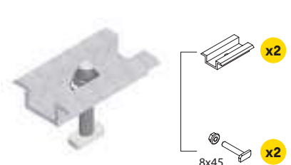
Grapa intermedia con tornillo
