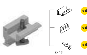
Grapa final con tornillo
