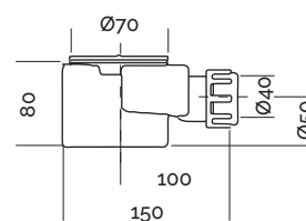
Desagüe estándar Ø 70 (mm)
