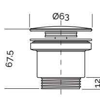
Válvula de salida libre Akron (mm)
