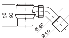
Desagüe estándar H98 (mm)
