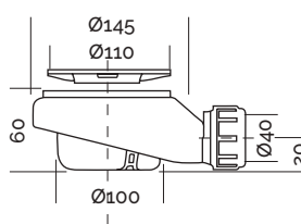
Desagüe extraplano (mm)
