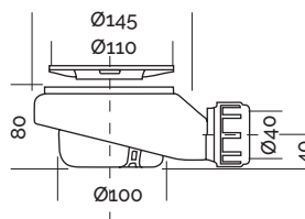
Desagüe estándar (mm)
