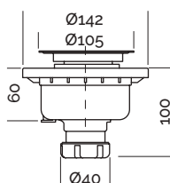
Desagüe vertical (mm)
