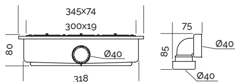
Desagüe line estándar (mm)
