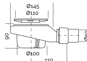
Desagüe de gran caudal (mm)
