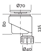
Desagüe vertical Ø 70 (mm)
