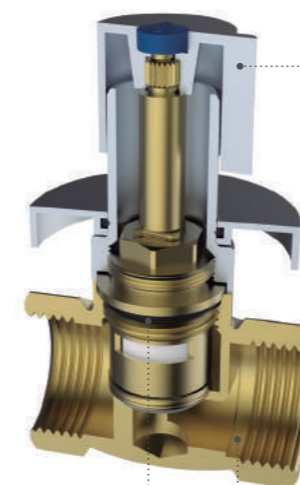
Junta de estanqueidad NBR
