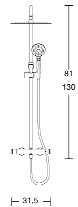
Fonte columna ducha termostático
